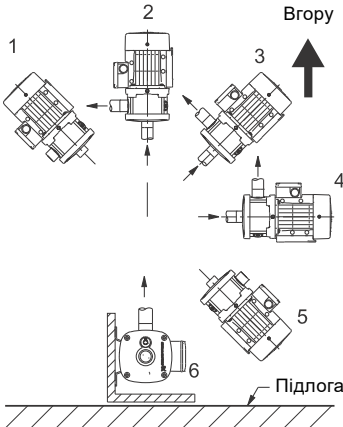
Рис. 1 Положення насоса
