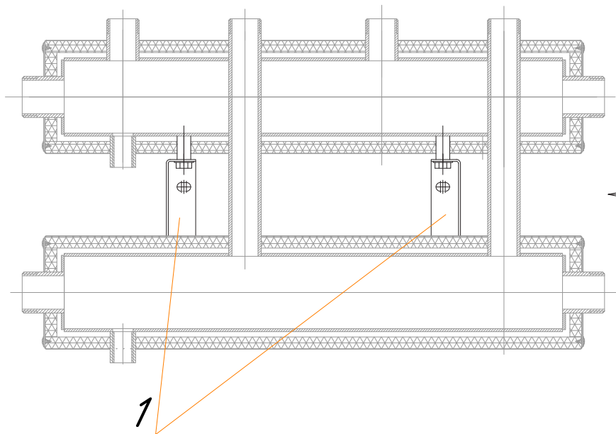
Схема колектора, встановленого на кронштейнах
