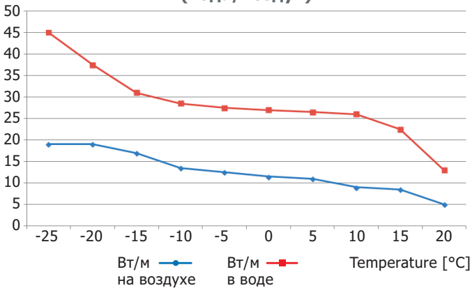
Выходная мощность при данной температуре (вода/воздух)
