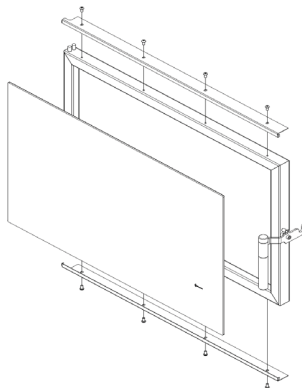
15. Схема заміни скла «JUNO». / Schemat wymiany szyby JUNO. / The JUNO glass-replacement diagram
