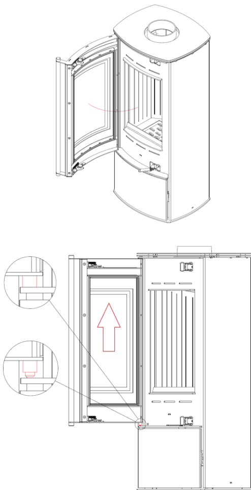
28. Схема заміни дверей у моделі «ATLAS». / Schemat wymiany drzwi ATLAS. / The ATLAS door-replacement diagram
