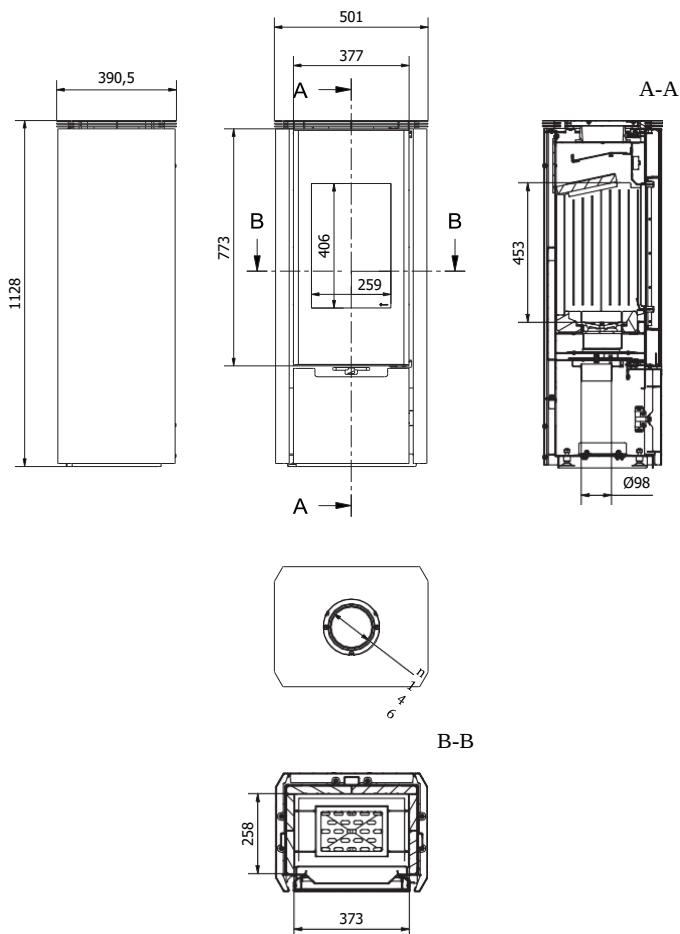
38. Креслення печі «ENYO» із зазначенням розмірів. / Zwymiarowany rysunek pieca ENYO. / Dimensioned Figure of the ENYO Stove.
