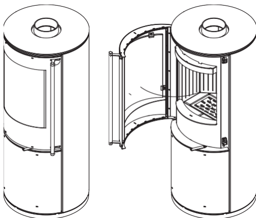
46. Схема заміни дверей в моделі «PICARD». / Schemat wymiany drzwi PICARD. / The PICARD door-replacement diagram.
