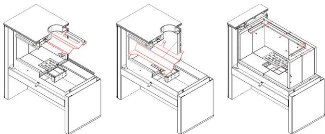
16. Схема заміни дверей «JUNO». / Schemat wymiany drzwi JUNO / The JUNO door-replacement diagram
