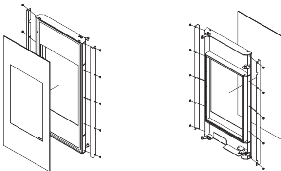
40. Схема заміни дверей в моделі «ENYO». / Schemat wymiany drzwi ENYO. / The ENYO door-replacement diagram.
