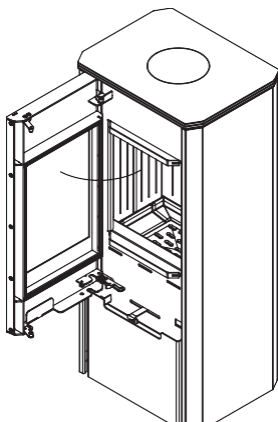
40. Схема заміни дверей в моделі «ENYO». / Schemat wymiany drzwi ENYO. / The ENYO door-replacement diagram.
