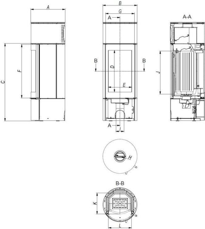
30. Розмірне креслення печі «ANTARES». / Zwymiarowany rysunek pieca ANTARES. / Dimensioned Figure of the ANTARES Stove.
