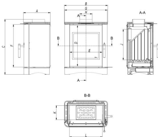
34. Креслення печі «VEGA» із зазначенням розмірів. Zwymiarowany rysunek pieca VEGA. Dimensioned Figure of the VEGA Stove.
