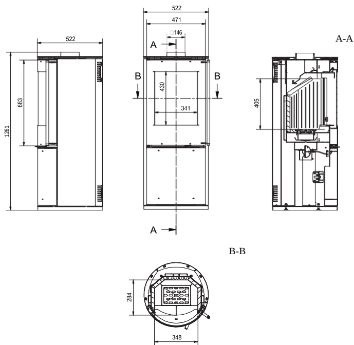
44. Креслення печі «PICARD». / Zwymiarowany rysunek pieca PICARD. / Dimensioned Figure of the PICARD Stove.
