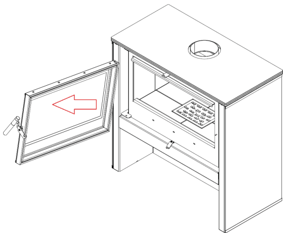
16. Схема заміни дверей «JUNO». / Schemat wymiany drzwi JUNO / The JUNO door-replacement diagram
