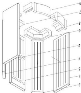
ПОСЛІДОВНІСТЬ ВІЙМАННЯ ЕЛЕМЕНТІВ АСКУМОТЕ (АККУМОТ) / KOLEJNOŚĆ WYIMANIA ELEMENTÓW ASKUМОTE
