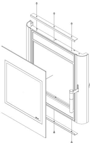
35. Схема заміни скла в печі «VEGA». / Schemat wymiany szyby w piecu VEGA. The VEGA glass-replacement diagram
