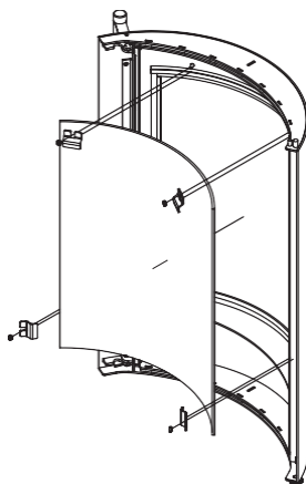
46. Схема заміни дверей в моделі «PICARD». / Schemat wymiany drzwi PICARD. / The PICARD door-replacement diagram.
