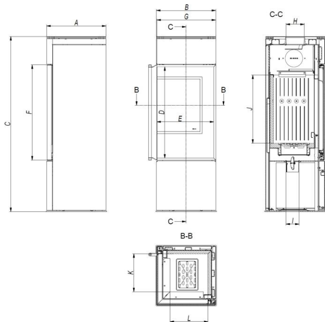
16. Схема заміни дверей «THOR». / Schemat wymiany drzwi THOR. / The THOR door-replacement diagram
