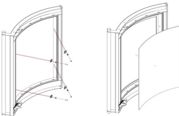
23. Схема заміни скла в печі «FALCON». / Schemat wymiany szyby w piecu FALCON / The FALCON glass-replacement diagram
