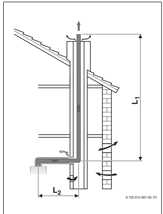
Мал. 9 Відведення димових газів у шахті згідно з B 33
