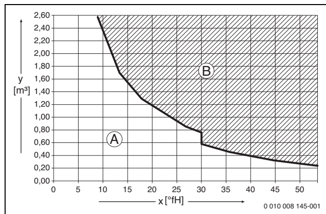
Мал. 20 Вимоги до води для заповнення та підживлення в °fH для приладів потужністю < 50 кВт
