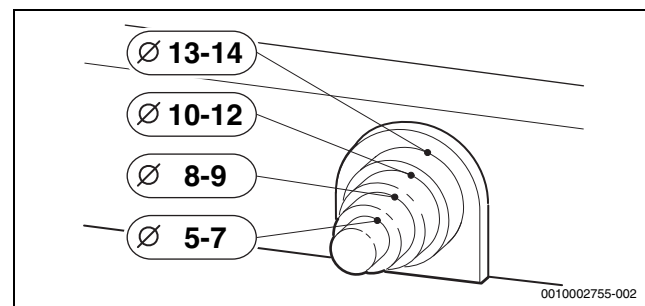
Мал. 31 Підгонка фіксатора проводу до діаметра кабелю
