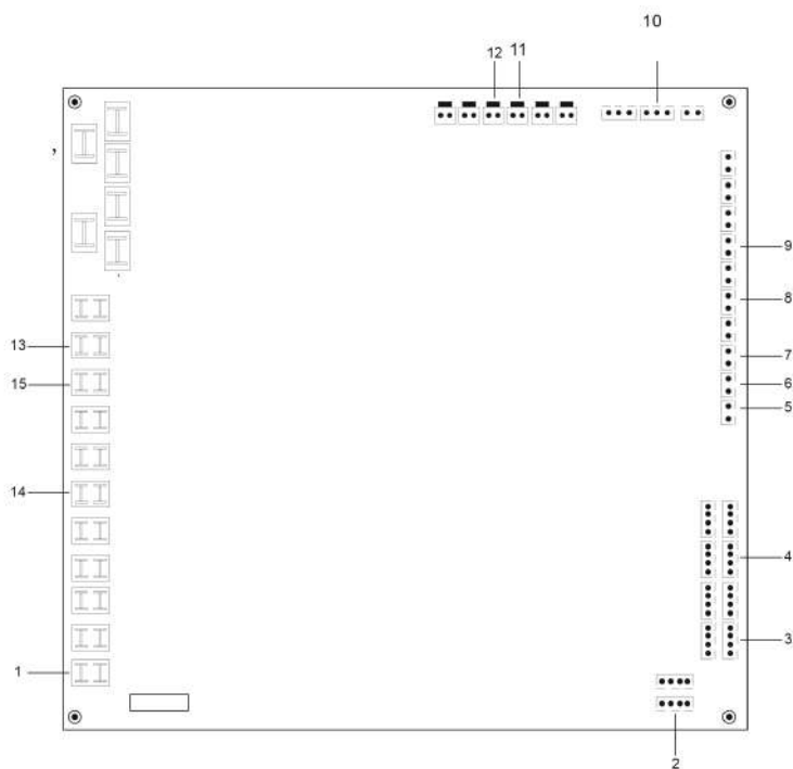
Мал.23 Плата внутрішніх блоків 14-16кВт, керування хладагентом
