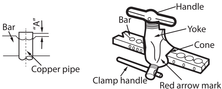
Мал.55 Інструмент для розвальцьовки труби
