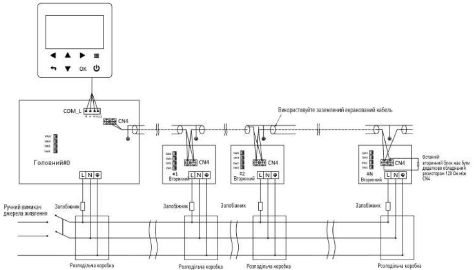
Мал.65 Схеми під'єднання кабелів каска
