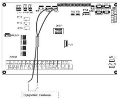
Мал.37 З'єднання для віддаленого вимкнення
