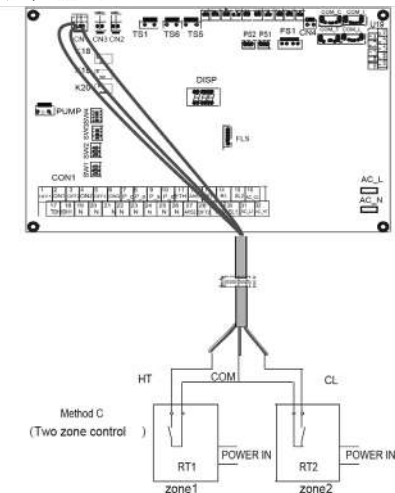
Мал.44 Метод 3.3'єднання двухзонний контроль режиму контролю
