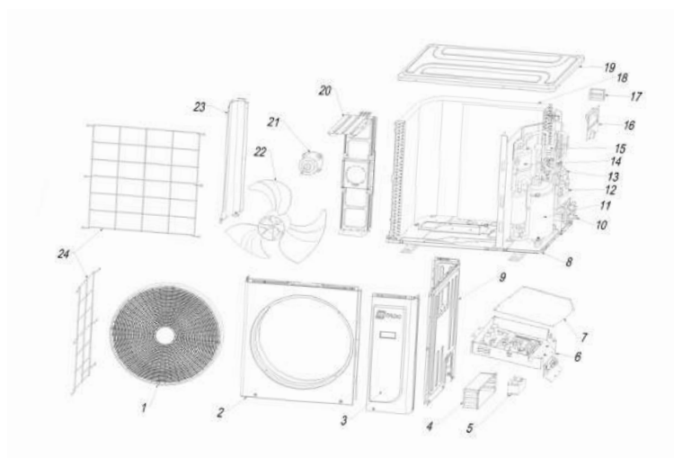
Мал.9 Схема структури зовнішнього блоку: 10-12 кВт (1-фазний)
