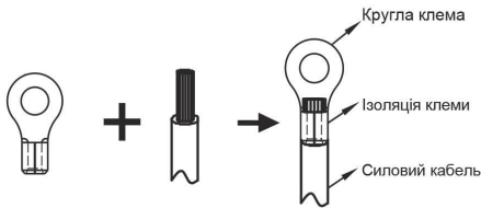
Мал. 31 Обжим круглої клема
