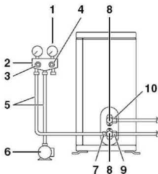
Мал.61 Схема використання обладнання для заправки фреоном
