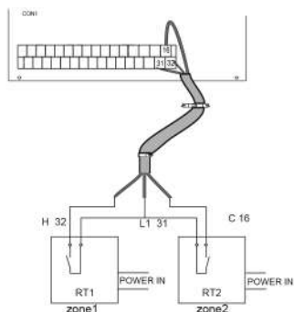
Мал.41 Метод С (Двוזонний контроль)
