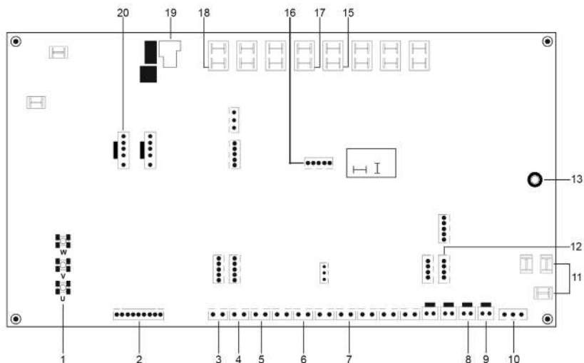
Мал.21 Плата внутрішніх блоків 8-10-12кВт, керування приводами та хладогентом
