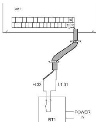
Мал.40. Схема Метод В (Однозонний контроль)
